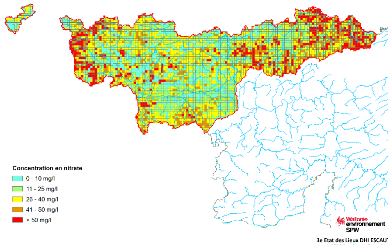
Figure 18 : Concentration en nitrate dans les eaux de lessivage au sommet de la nappe de base pour la période 2012-2016 (EPICgrid, 2016)
