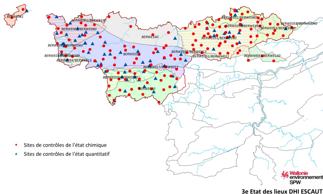
Figure 5 : Réseau de surveillance des masses d'eau souterraine du district de l'Escaut - Source : DGO3, DESo (2009-2013)
