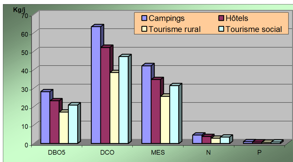
Graphique 2.2.2/2 : charge polluante générée (Kg/j) dans le sous-bassin Escaut-Lys, en fonction du service pour chacun des paramètres composant l'EH.
