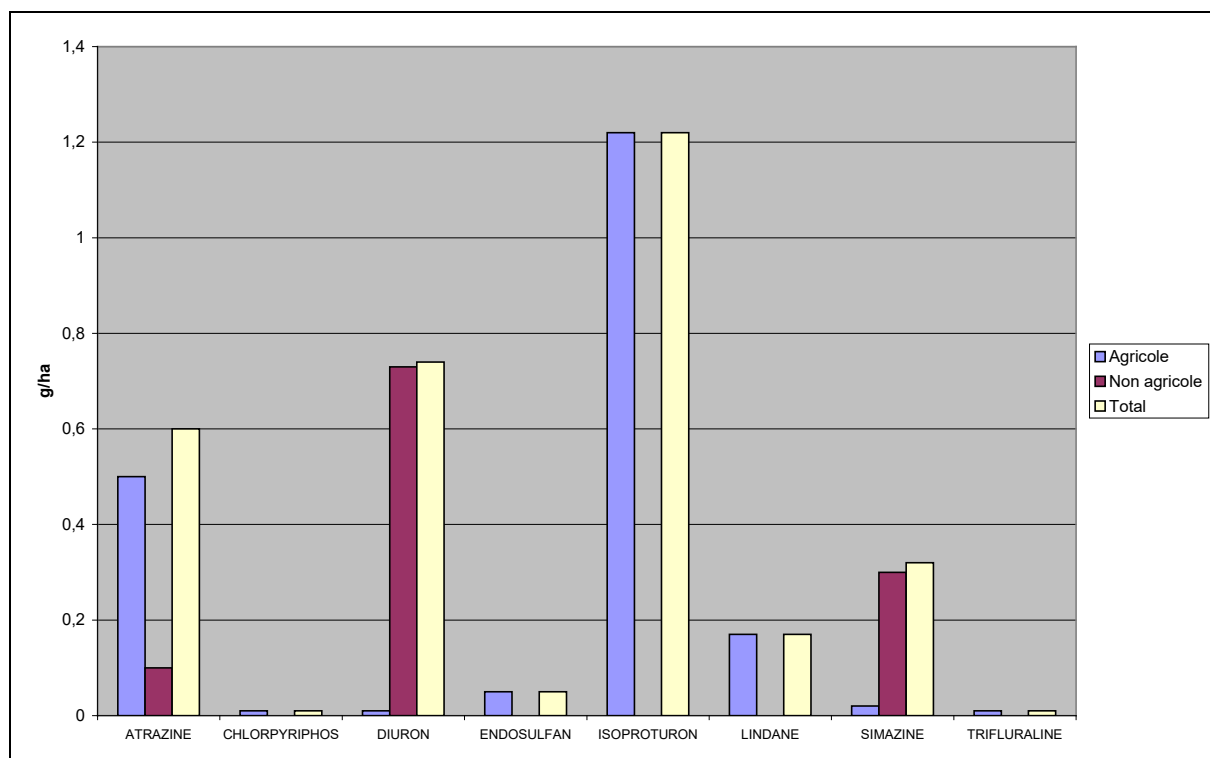
Graphique 2.2.4/4: Emissions des pesticides prioritaires vers les eaux de surface. Sous-bassin de l'Escaut-Lys (année 2000).
