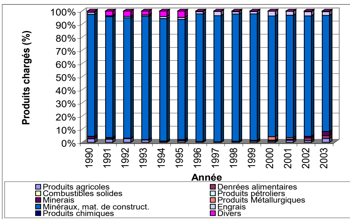
Graphique 2.2.9.5/2 : types de produits chargés entre 1990 et 2003 sur les différentes voies d'eau traversant le sous-bassin Escaut-Lys.
