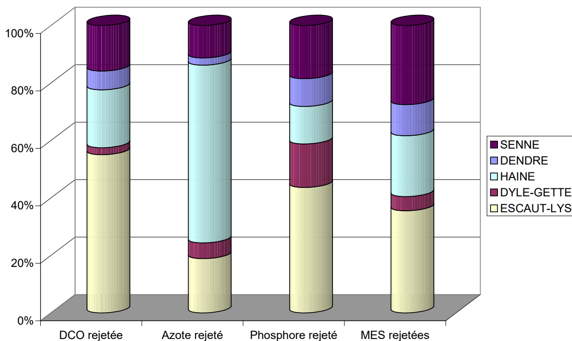
Graphique 2.2.3/3 : importance de la charge industrielle en DCO, azote, phosphore et matières en suspension (MES) rejetée dans le sous-bassin Escaut-Lys par rapport aux autres sous-bassins de la partie wallonne du District Hydrographique de l'Escaut.
