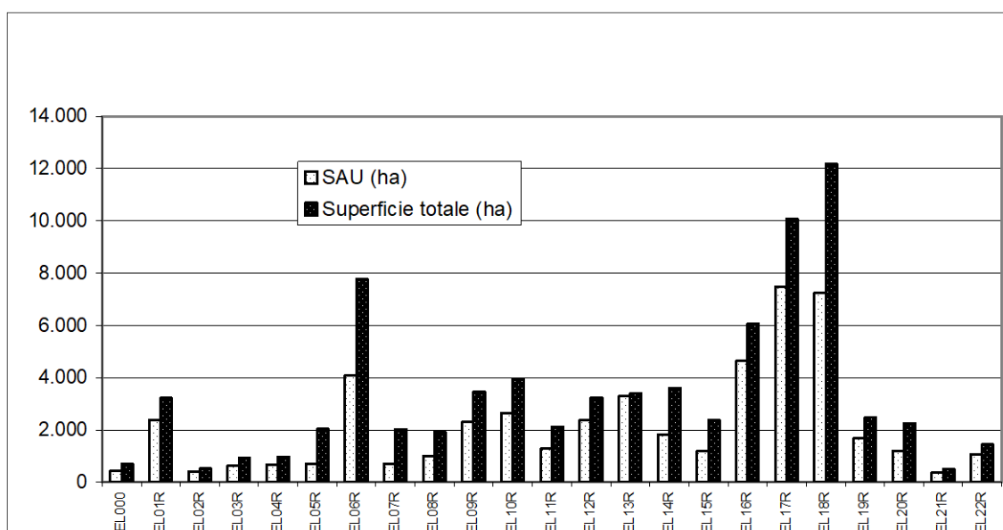
Graphique 2.2.4/2 : surface agricole utile (SAU en ha) par masse d'eau dans le sous-bassin Escaut-Lys. (année 2000)
