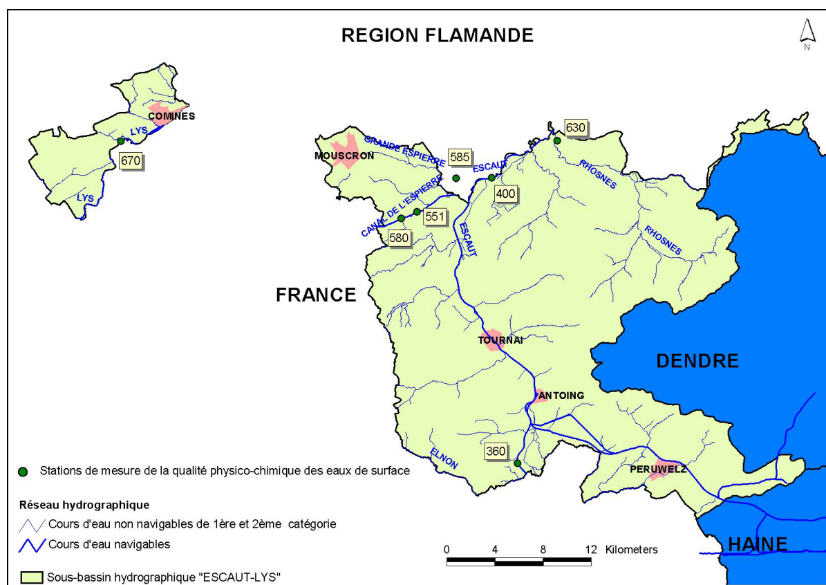
Carte 2.3.2/1 : Localisation des points d'échantillonnage du réseau physico-chimique dans le sous-bassin hydrographique "Escaut-Lys" en 2002.
