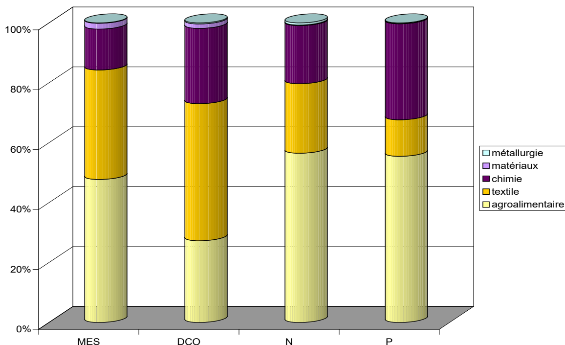
Graphique 2.2.3/2 : répartition de la charge en DCO, azote, phosphore et matières en suspension (MES) rejetée dans le sous-bassin Escaut-Lys en fonction des principaux secteurs industriels.
