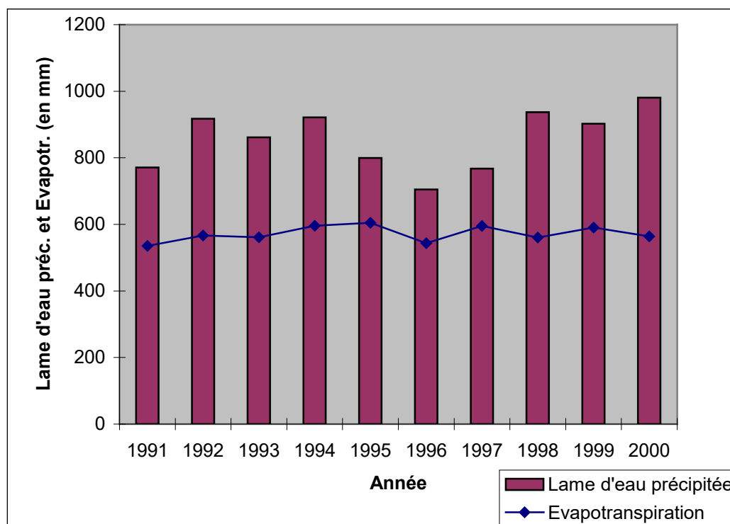
Graphique 1.2/1 : lame d'eau précipitée et évapotranspiration pour le sous-bassin Escaut-Lys (bassin de l'Escaut).
