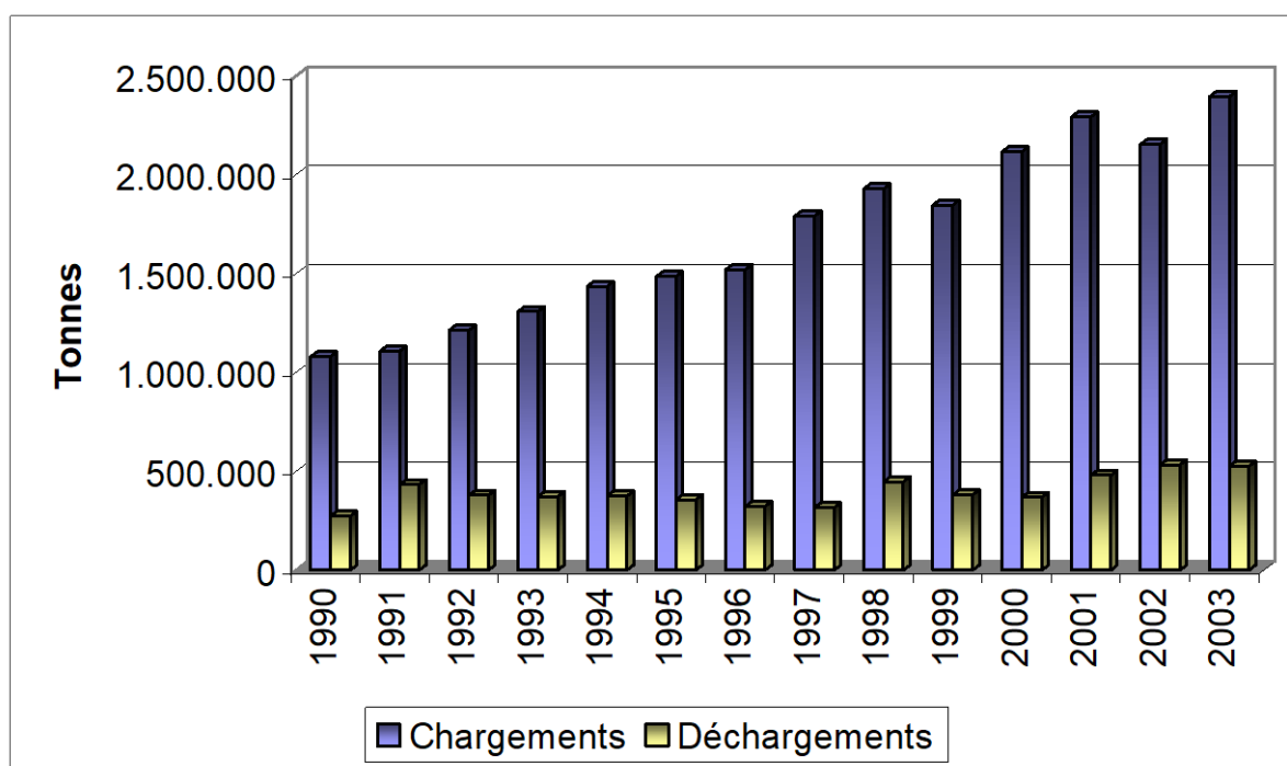
Graphique 2.2.9.5/1 : évolution des tonnages chargés et déchargés entre 1990 et 2003 sur les différentes voies d'eau traversant le sous-bassin Escaut-Lys.
