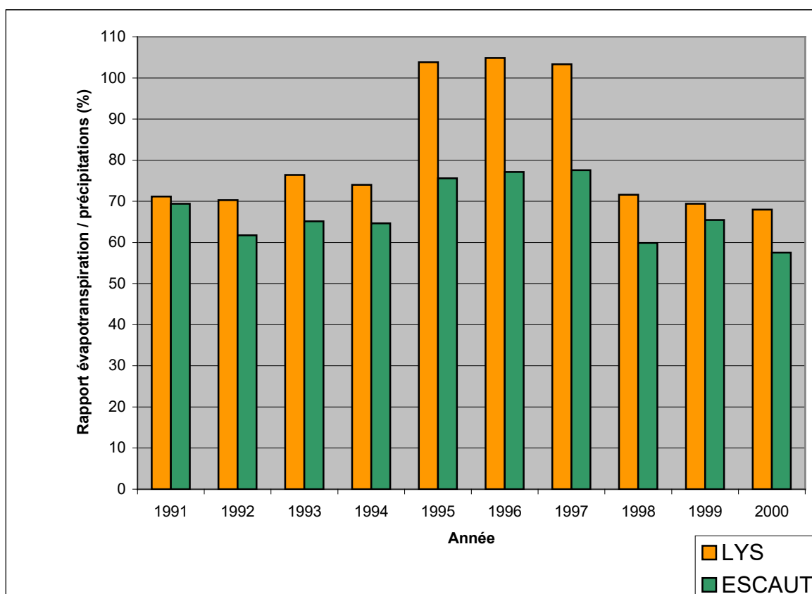
Graphique 1.2/3 : rapport évapotranspiration / précipitations pour le sous-bassin Escaut-Lys.
