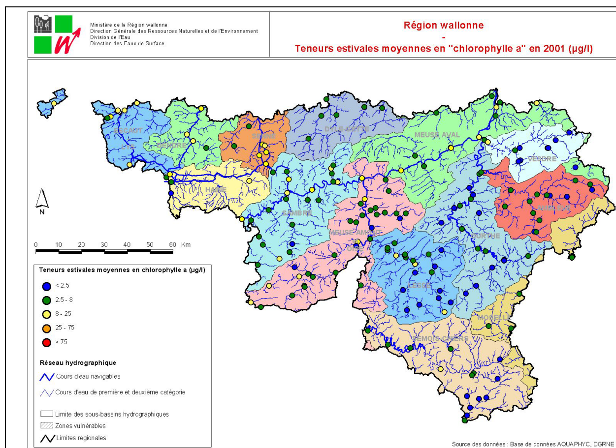
Carte 2.3.2/3 : Teneurs estivales moyennes en "chlorophylle a" en 2001 sur les cours d'eau wallons. Source : Base de données AQUAPHYC, DGRNE, 2003
