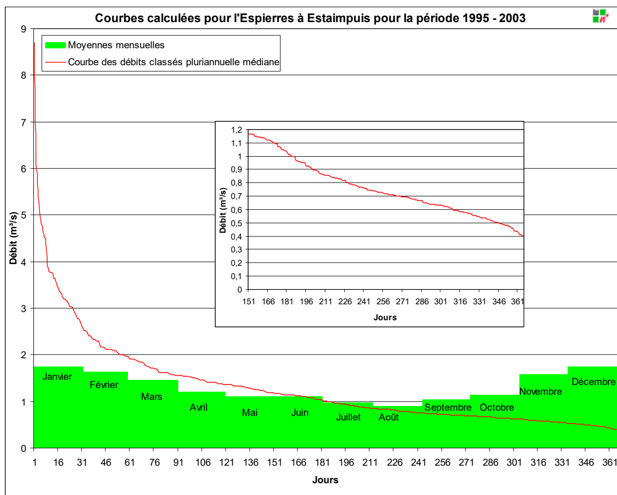
Graphique 2.3.1/2 : Courbe des débits classés pluriannuelle médiane et moyennes mensuelles interannuelles de l'Espierres à Estaimpuis pour la période 1995 - 2003 (sous-bassin de Escaut - Lys).
