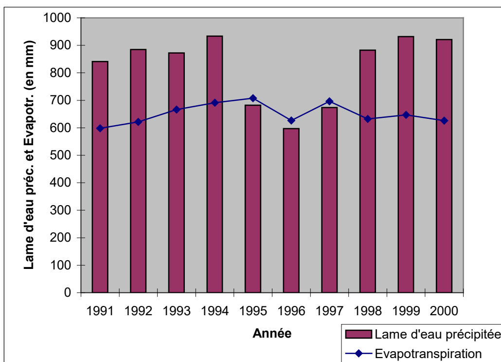
Graphique 1.2/2 : lame d'eau précipitée et évapotranspiration pour le sous-bassin Escaut-Lys (bassin de la Lys).
