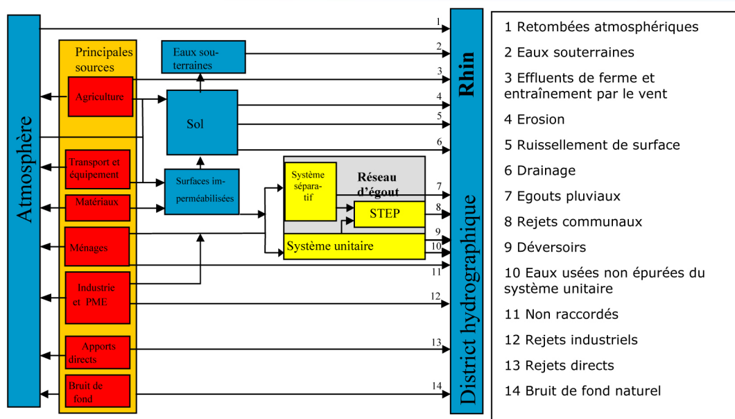
Figure 2 : voies d'apport définies pour la détermination des pressions sur les eaux de surface
