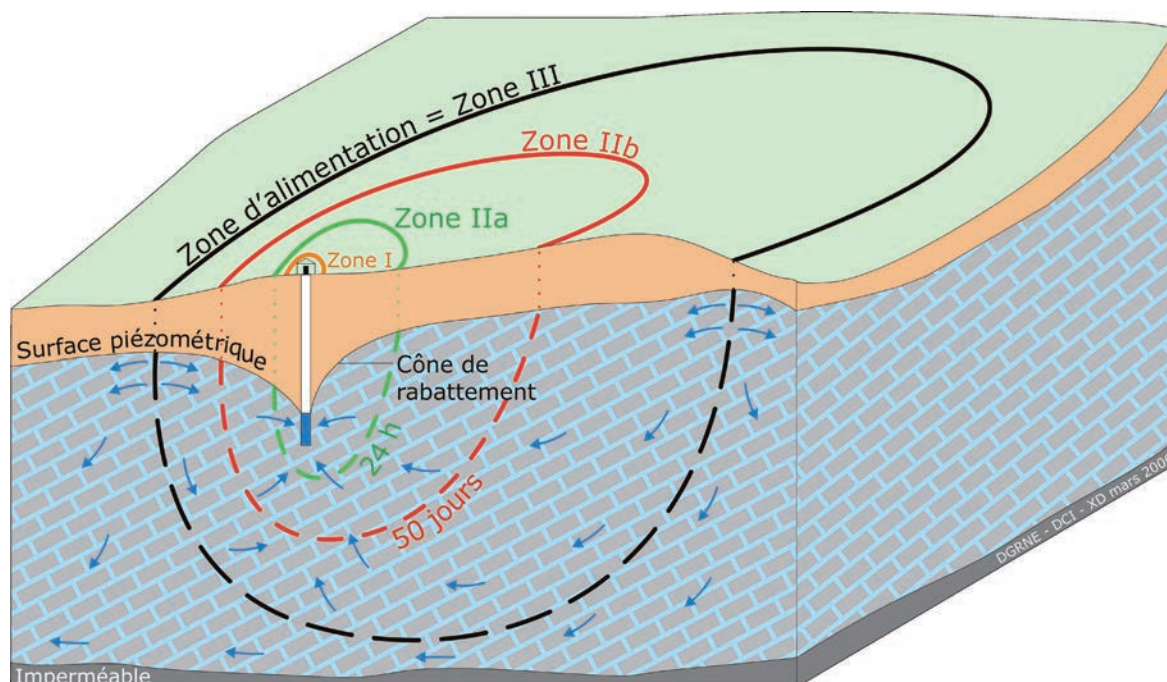
Figure 16: Les différents périmètres de protection d'un captage.
