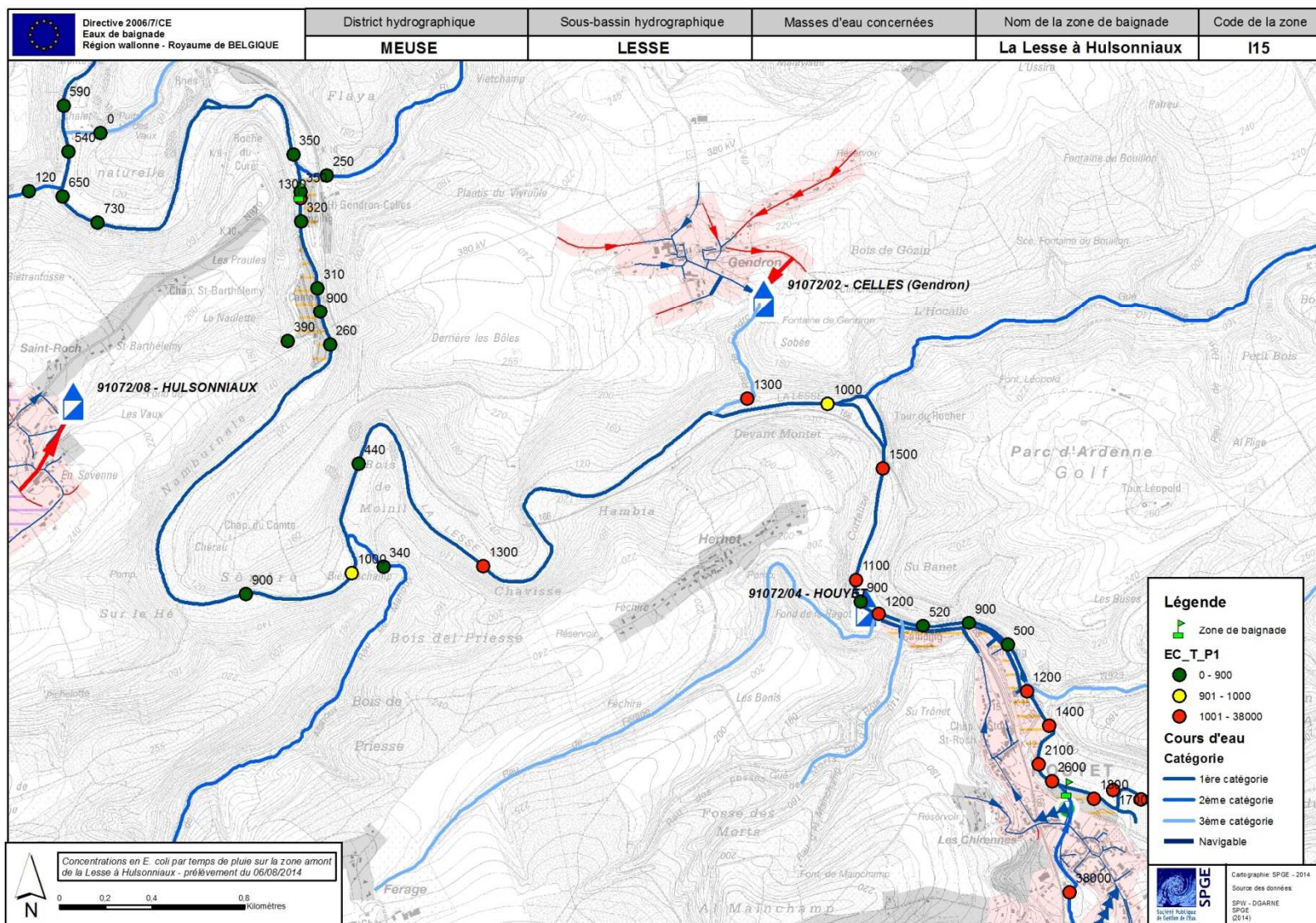
Figure 4: concentrations en E. coli (CFU/100ml) mesurées par temps de pluie le 06/08/14 à proximité de la zone de baignade.
