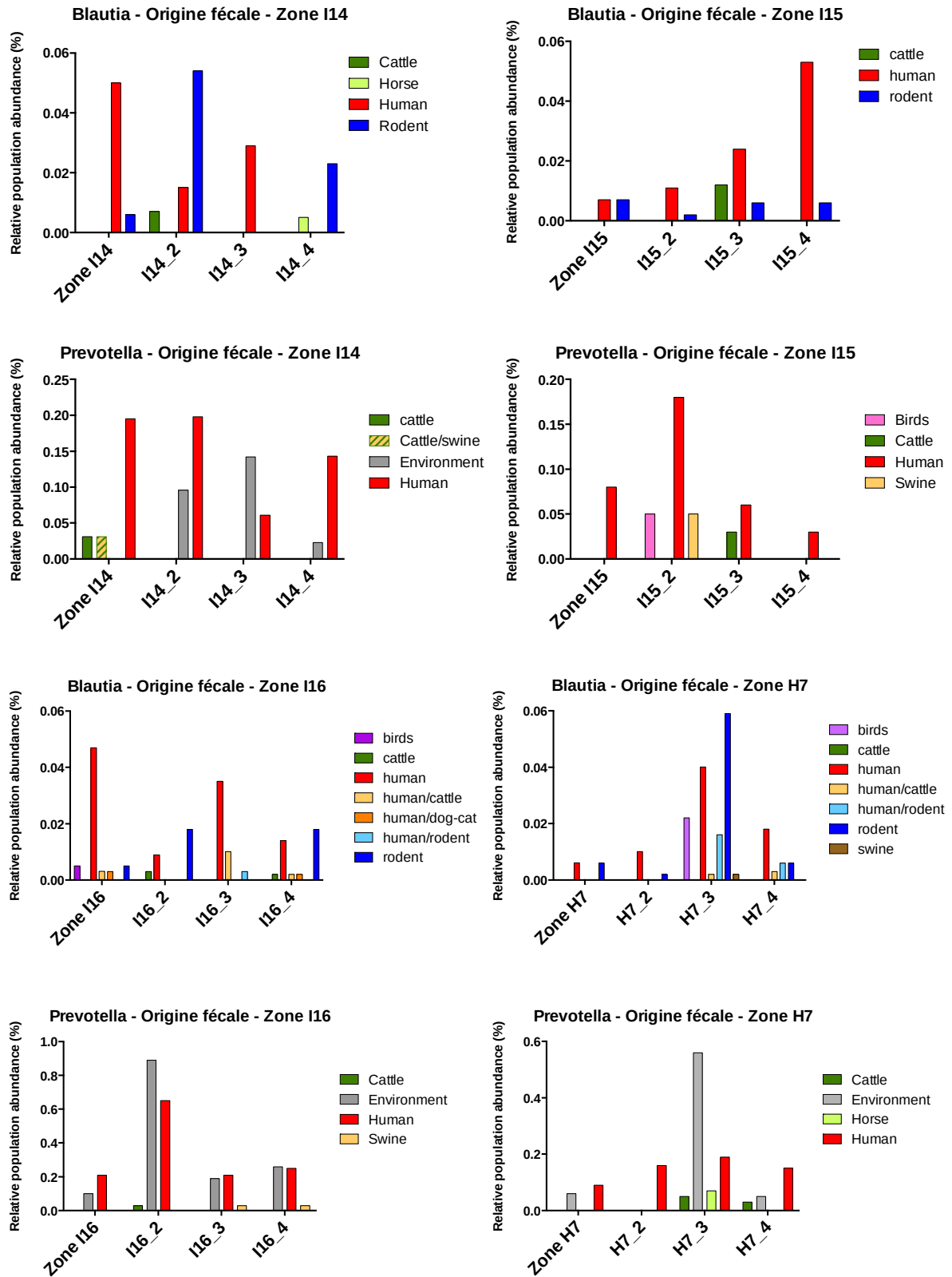
Figure 7: Recherche globale des indicateurs Blautia et Prevotella (source des données: SPW-DGO3-DESU, 2014).
