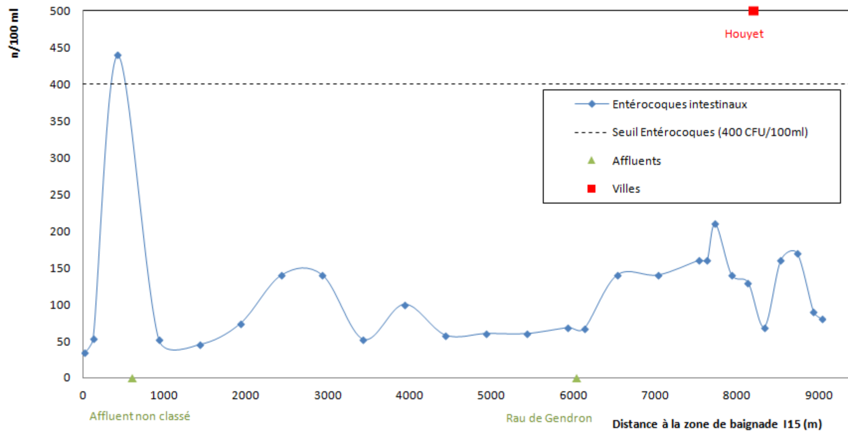
Figure 3: évolution spatiale des concentrations en entérocoques intestinaux en zone d'amont pour la zone I15
