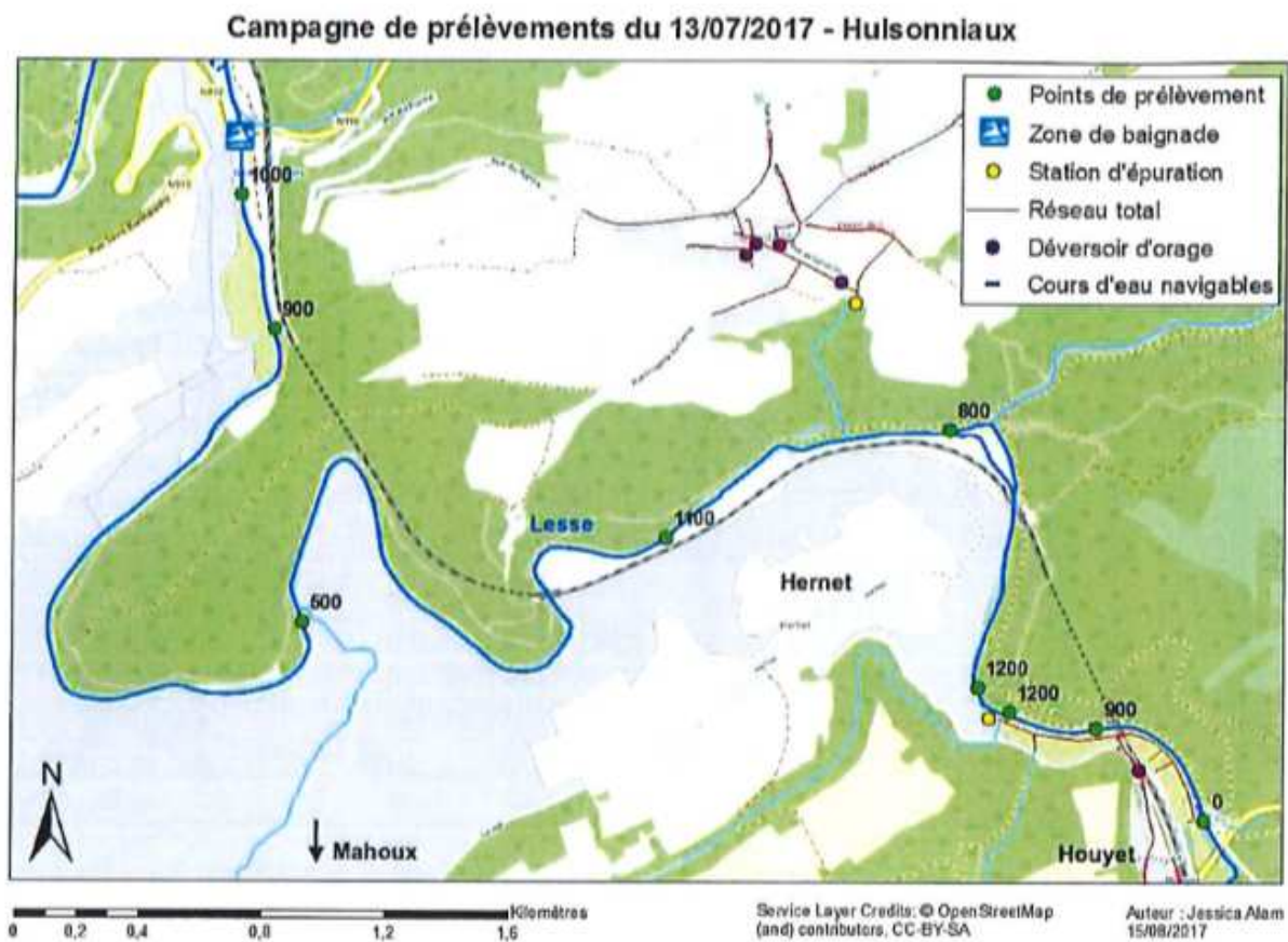
Figure 2 : campagne de prélèvement par temps de pluie réalisée sur la zone amont de Hulsonniaux, le 13/07/2017 (Source : « Contamination fécale en rivières, Etude de cas sur la Lesse et développement de traceurs génétiques équins », Jessica ALAM, UCL, 2017).
