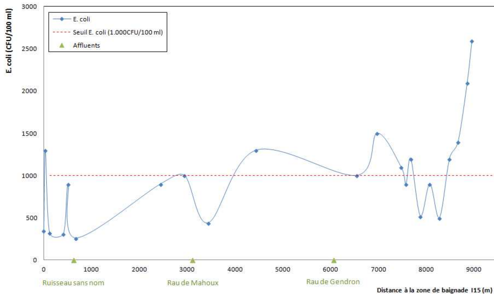
Figure 5: profil en long de l'évolution des concentrations en E. coli en amont de la zone de baignade I15 par temps de pluie (échantillons prélevés le 06/08/2014).
