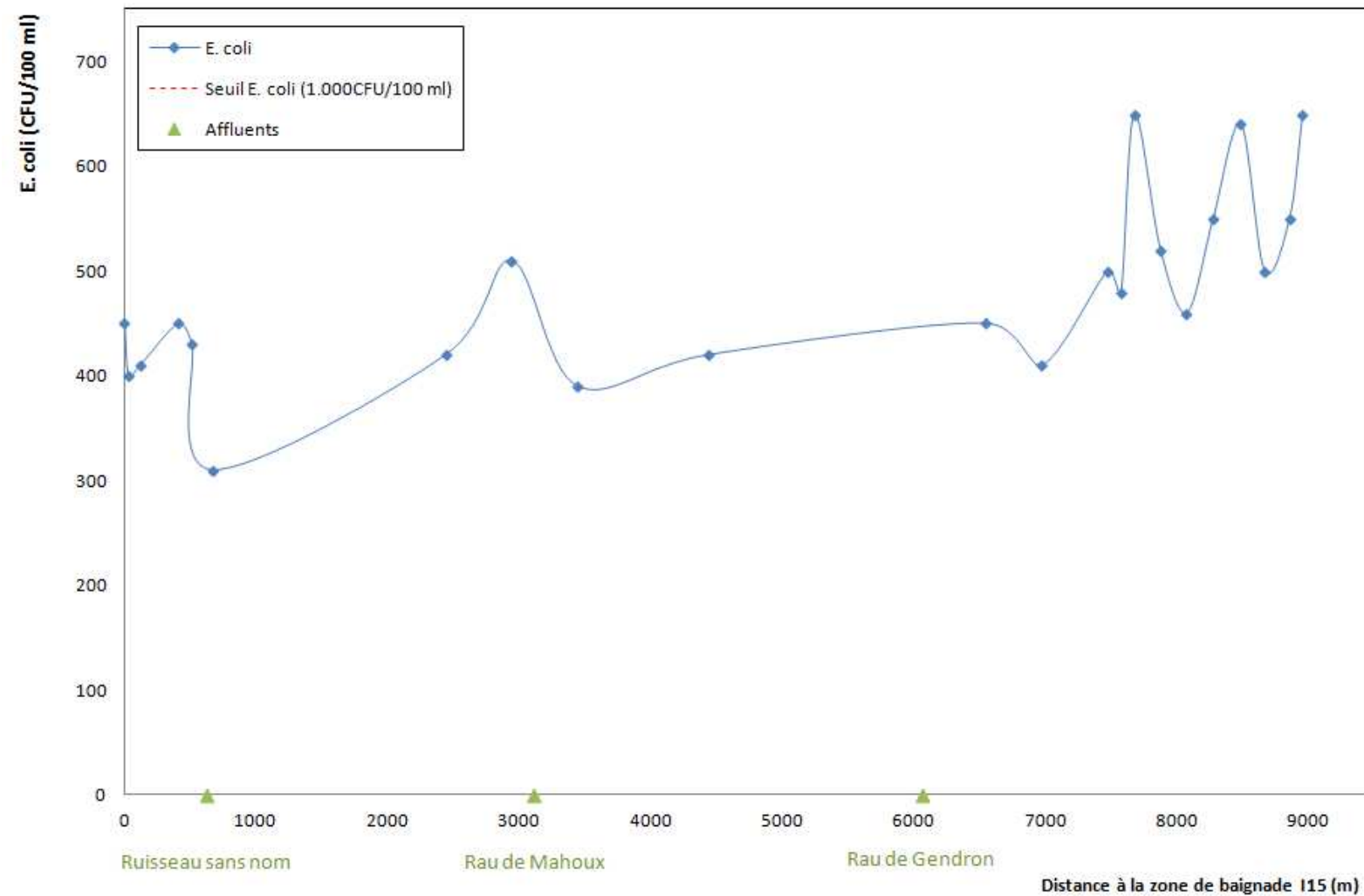
Figure 3: profil en long de l'évolution des concentrations en E. coli en amont de la zone de baignade I15 par temps sec (échantillons prélevés le 25/08/2014).
