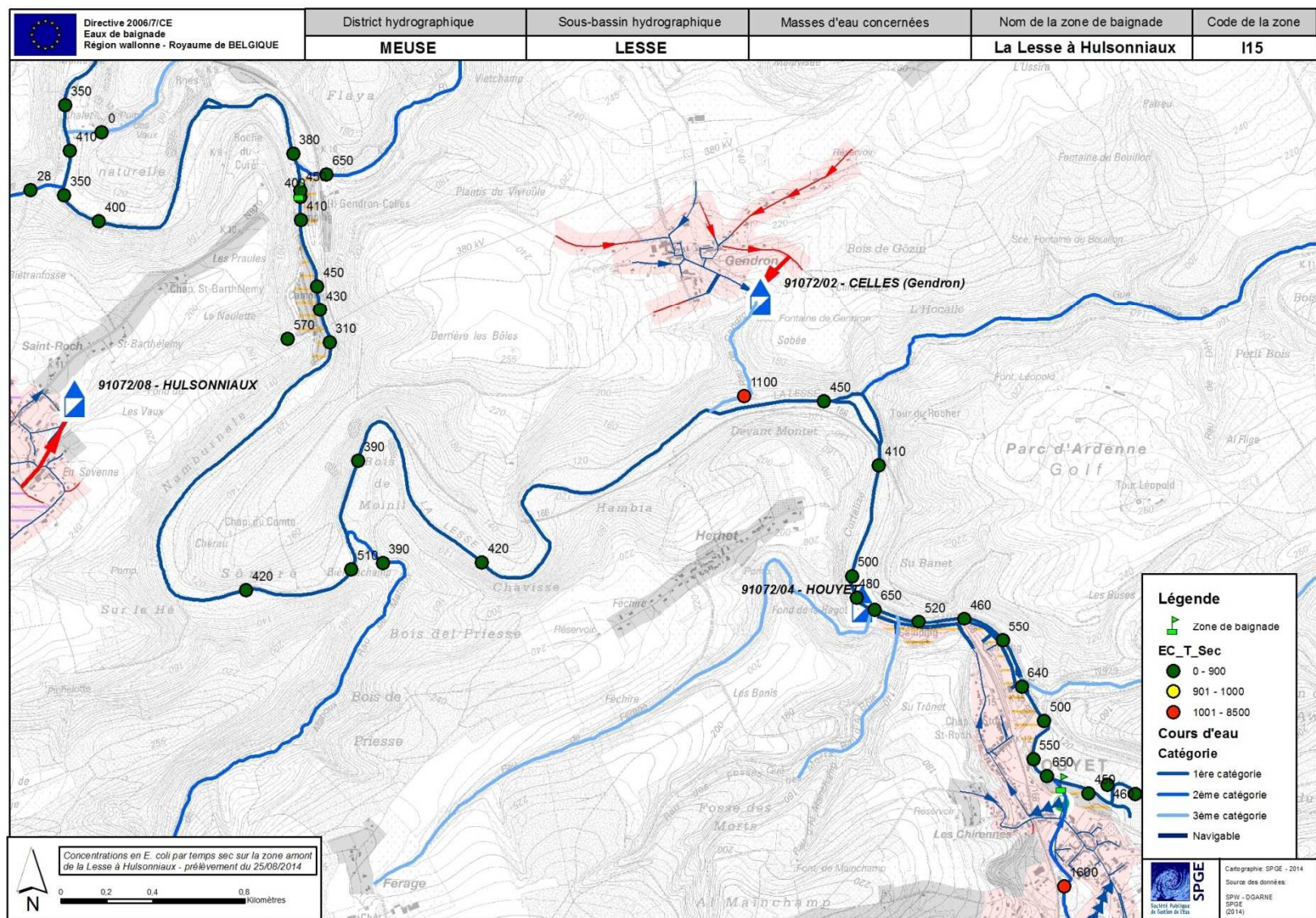
Figure 2: concentrations en E. coli (CFU/100ml) mesurées par temps sec le 25/08/14 à proximité de la zone de baignade.
