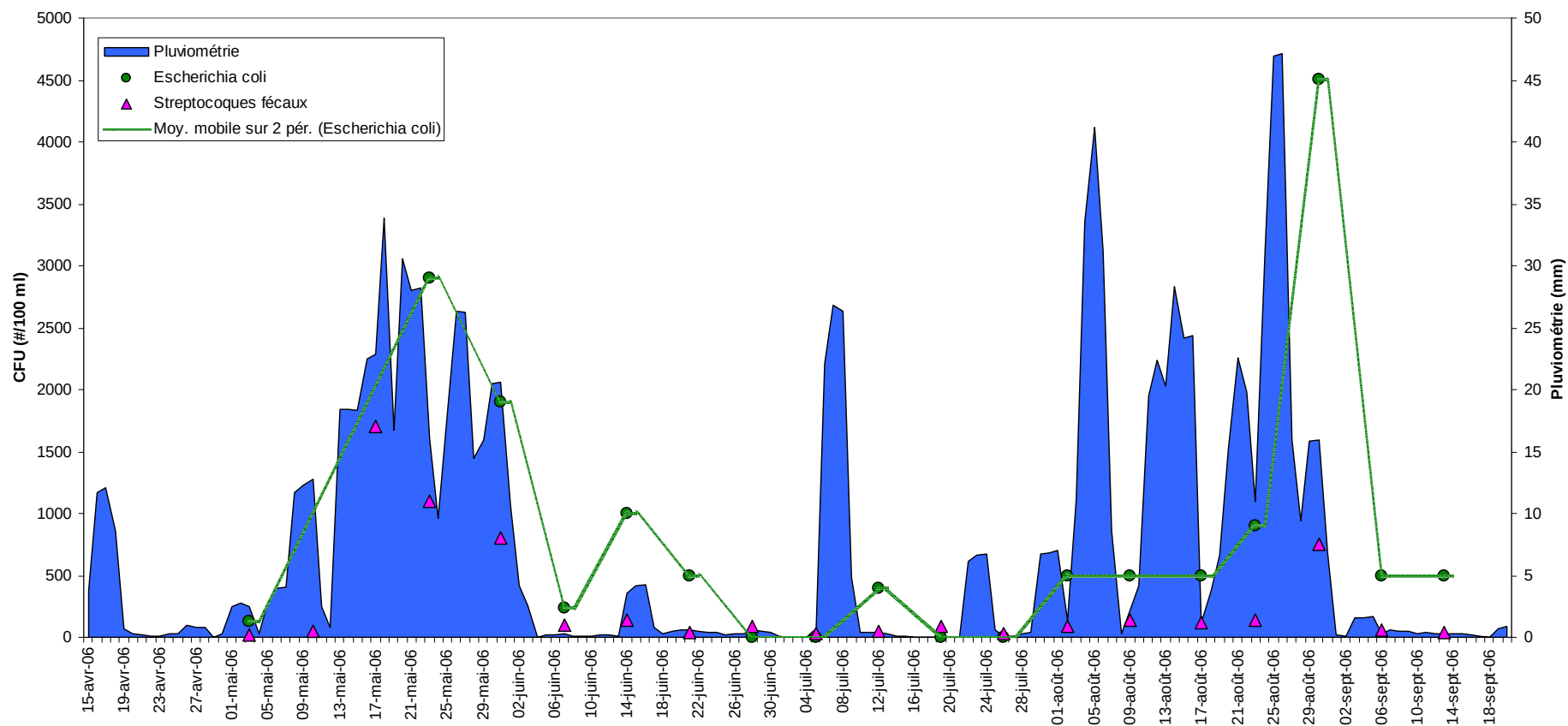
Figure 50 : évolution des paramètres bactériologiques et de la pluviométrie cumulée sur trois jours au cours de l'année 2006
