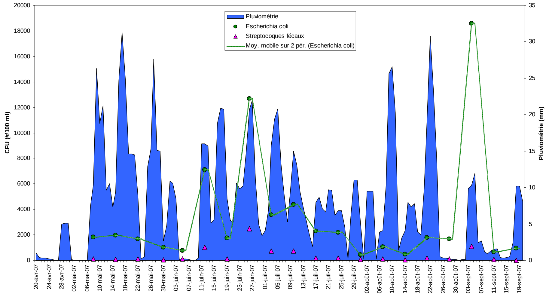
Figure 51: évolution des paramètres bactériologiques et de la pluviométrie cumulée sur trois jours au cours de l'année 2007.
