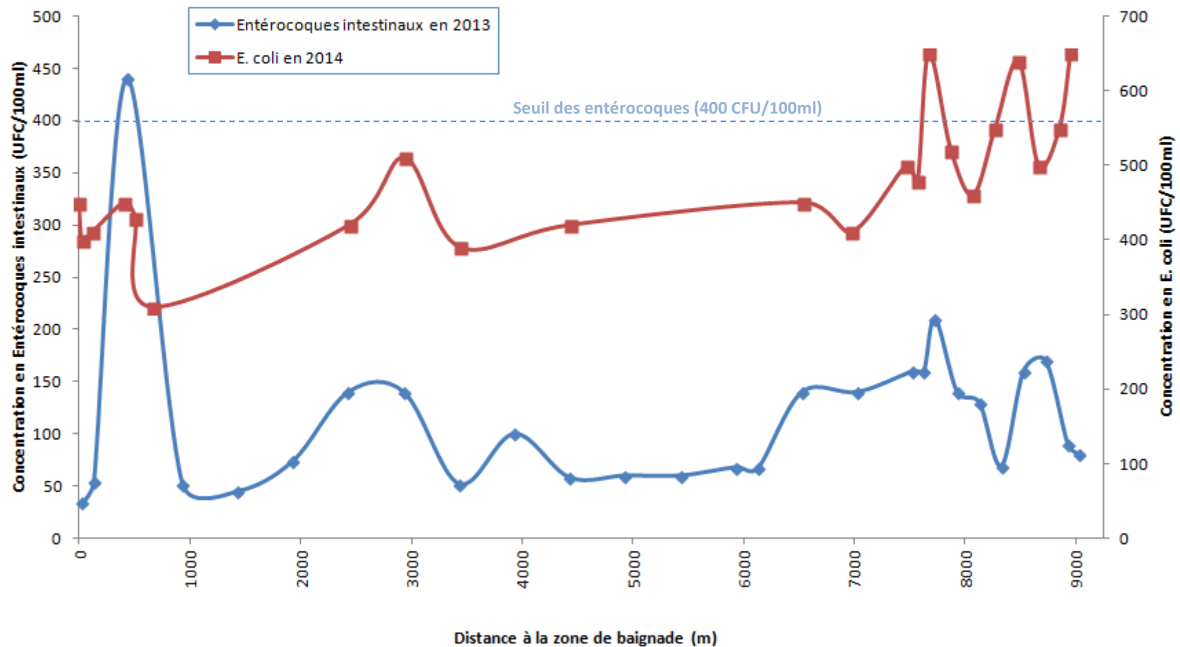
Figure 6: comparaison des résultats des prélèvements réalisés en 2013 et 2014 sur la zone amont de Hulsonniaux par temps sec.
