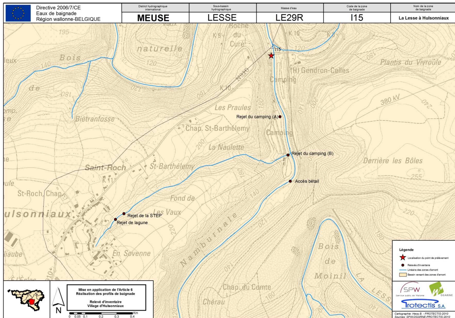
Figure 32: points noirs (= potentiel de dégradation de la qualité bactériologique du cours d'eau) relevés sur le terrain à proximité du village de Hulsonniaux. Source : PROTECTIS, 2010
