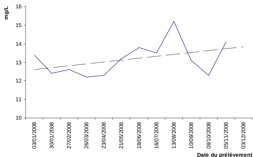
Figure 11: évolution des concentrations en sulfates ( \text{SO}_4^{2-} ) au cours de l'année 2008 pour la masse d'eau LE29R. Source des données : SPW/DGARNE, 2009
