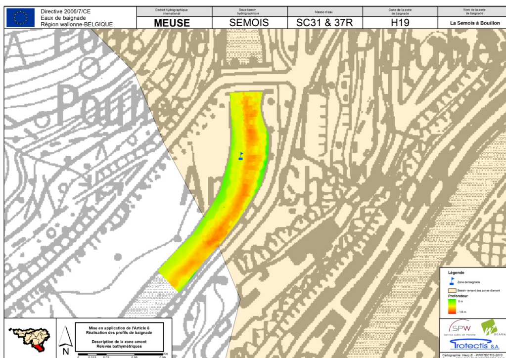
Figure 4 : relevés bathymétriques de la zone de baignade H19. Source des données : SPW/DGO2, 2010.
