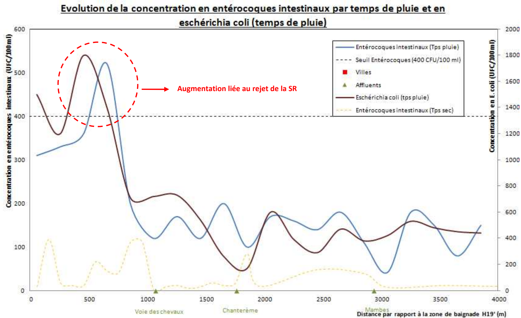
Figure 5: évolution des concentrations en entérocoques et E. coli au droit de chaque point de prélèvement réalisé par temps de pluie et comparaison avec les concentrations en entérocoques relevées par temps sec
