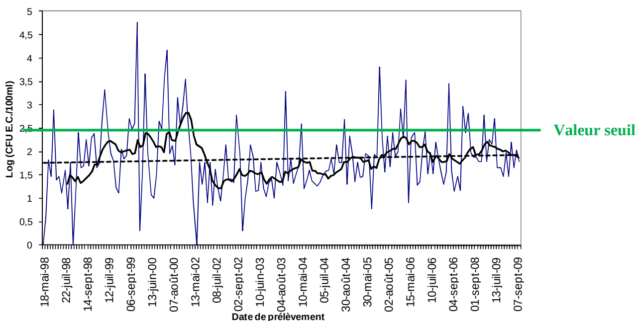
Figure 16: évolution des concentrations en Entérocoques intestinaux (Log) sur la zone de baignade H19 entre 1998 et 2009 (n=178). Source des données: SPW/DGARNE, 2010
