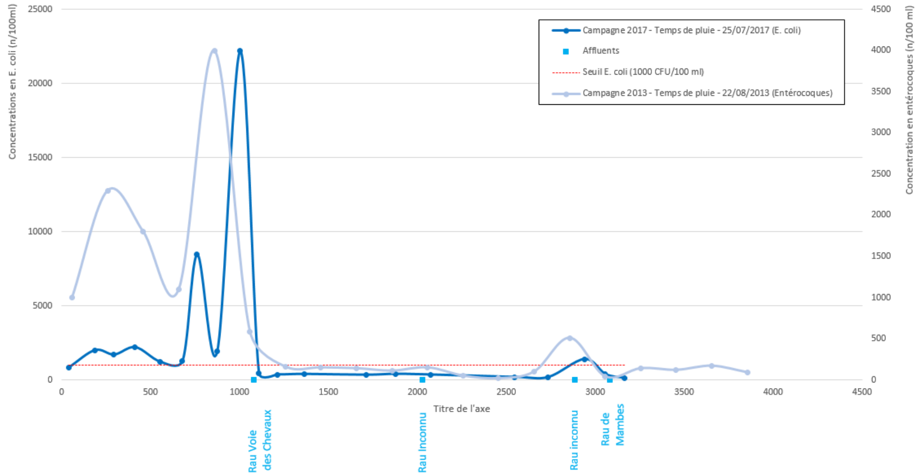
Figure 7: comparaison des épisodes "temps de pluie" de 2013 et 2017.
