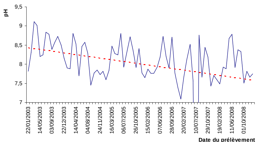
Figure 9: évolution du pH entre 2003 et 2008 pour la masse d'eau SC37R. Source des données : SPW/DGARNE, 2009
