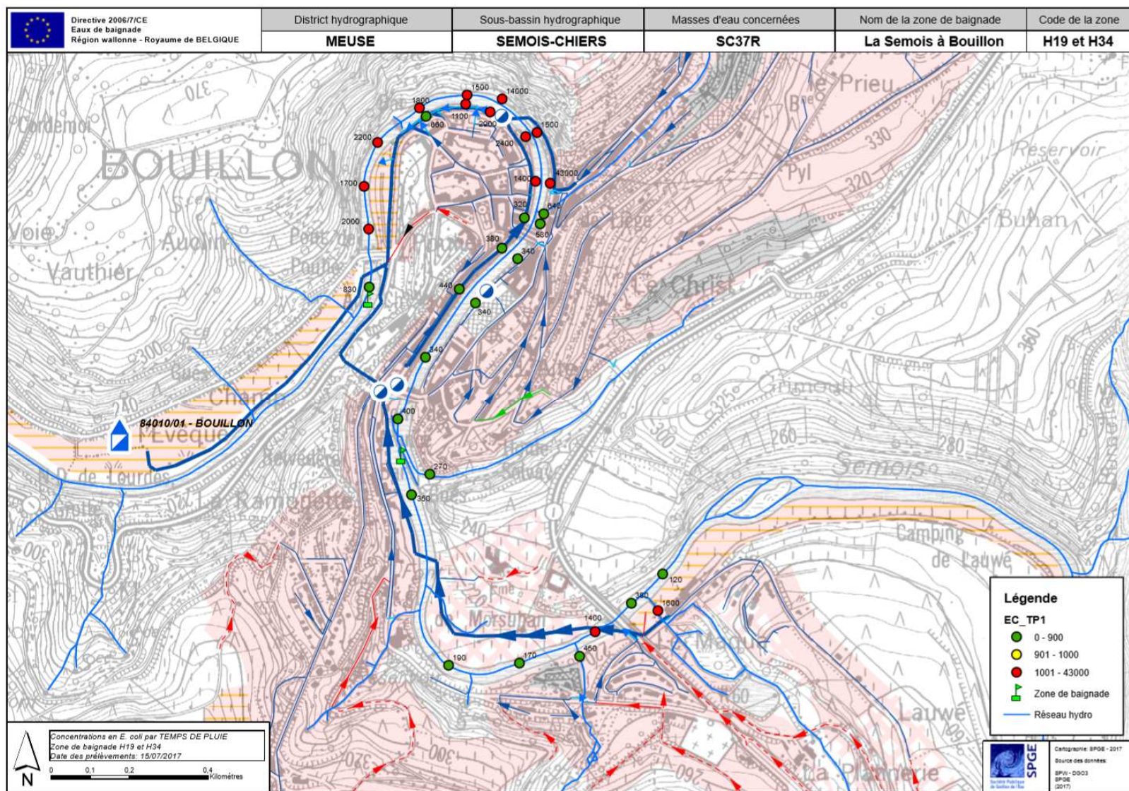
Figure 3 : localisation des points de prélèvement et concentrations en E. coli mesurées lors de la campagne « temps de pluie » du 25/07/2017 (Source des données : SPGE, 2017).
