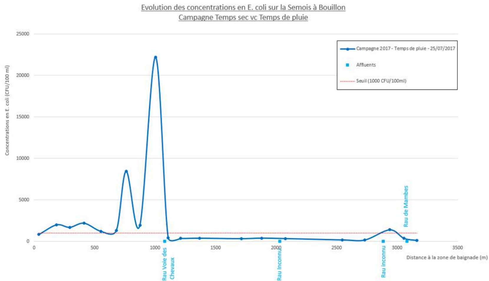
Figure 5 : profil longitudinal de l'évolution de la qualité bactériologique de la Semois sur la zone amont de Bouillon, lors de l'épisode « temps de pluie » du 25/07/2017. (Source des données : SPGE, 2017).
