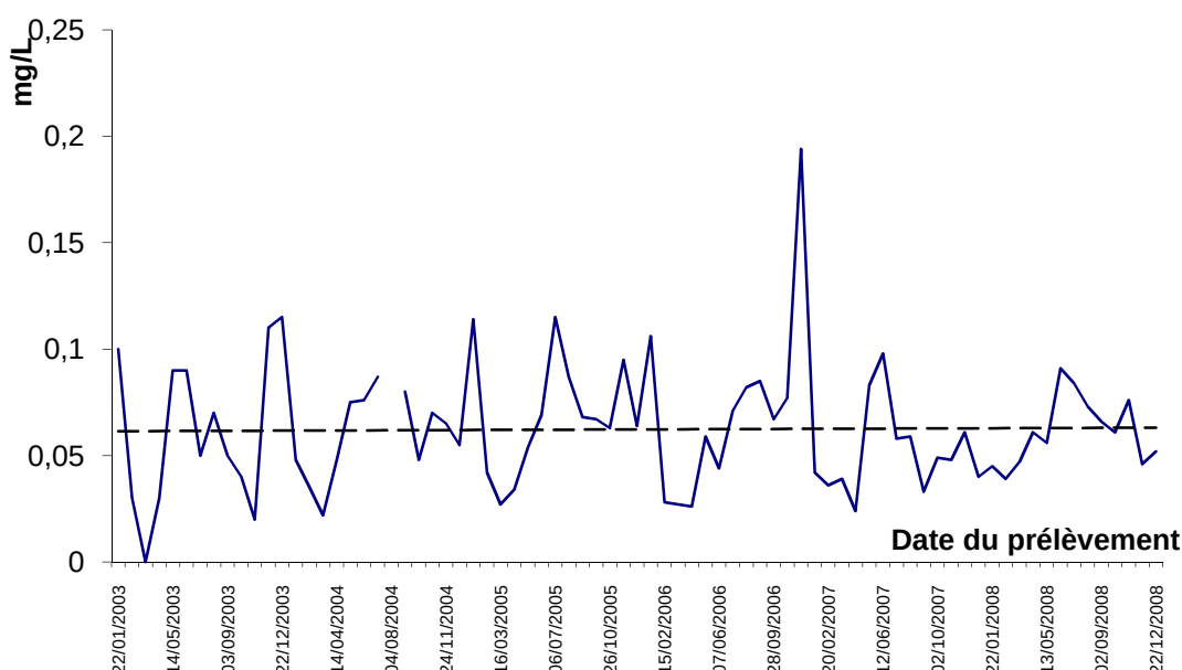
Figure 11 : évolution des concentrations en phosphore entre 2003 et 2008 pour la masse d'eau SC37R.
