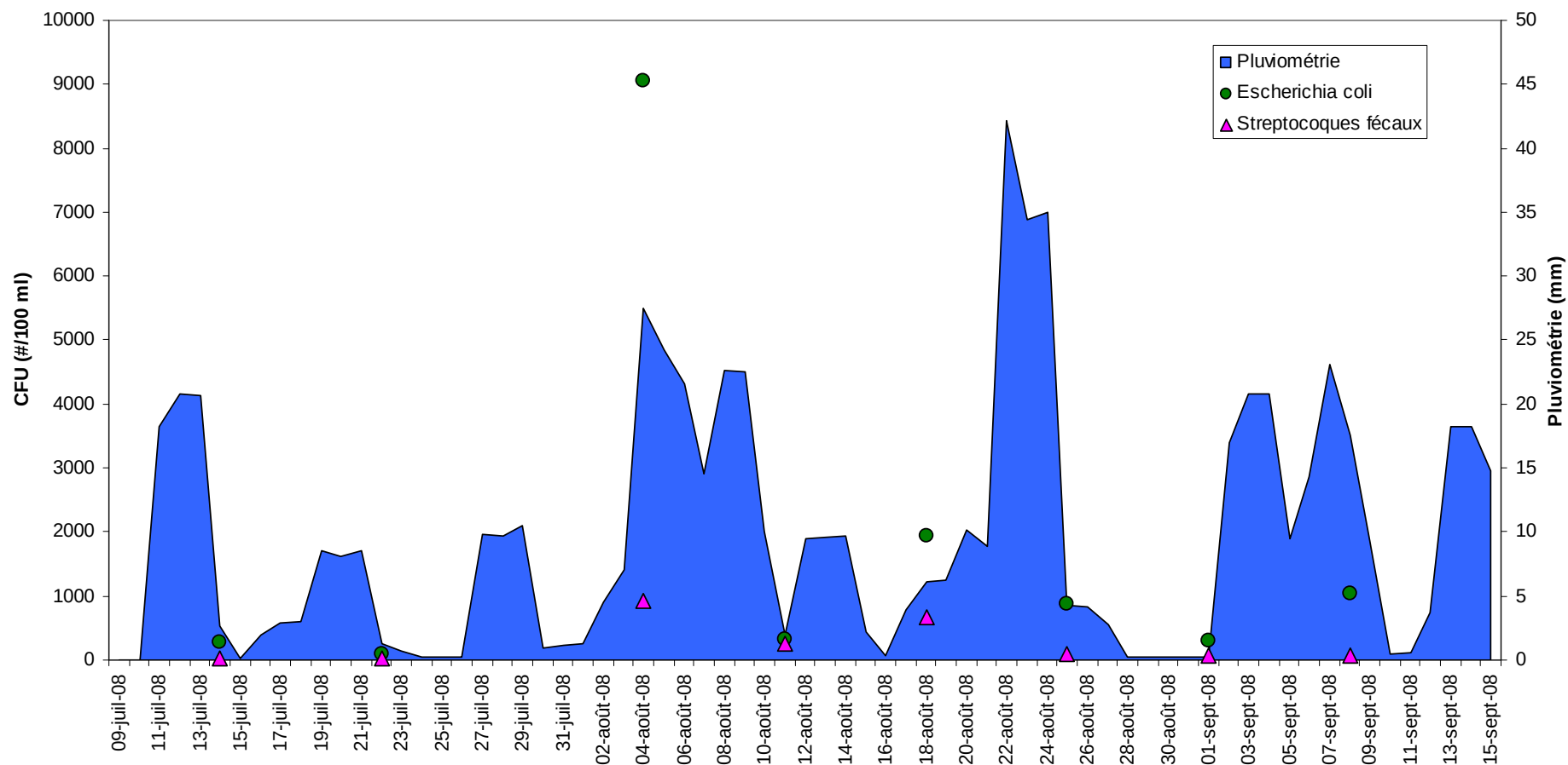
Figure 43 : évolution des paramètres bactériologiques et de la pluviométrie cumulée sur trois jours au cours de l'année 2008.
