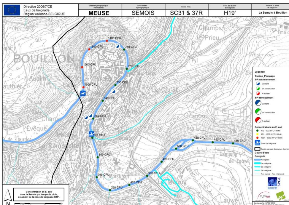
Figure 9: concentrations en E. coli relevées par temps de pluie et localisation des stations de relevage
