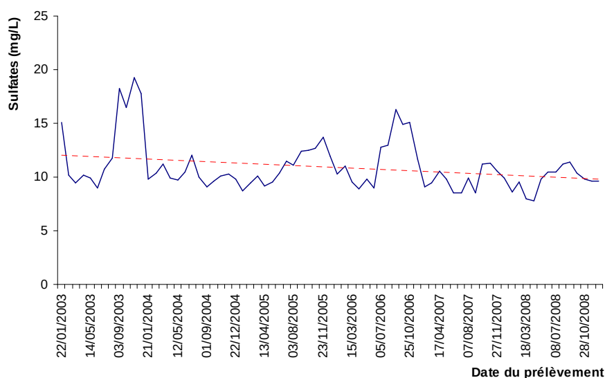
Figure 12: évolution des concentrations en sulfates entre 2003 et 2008 pour la masse d'eau SC37R. Source des données : SPW/DGARNE, 2009
