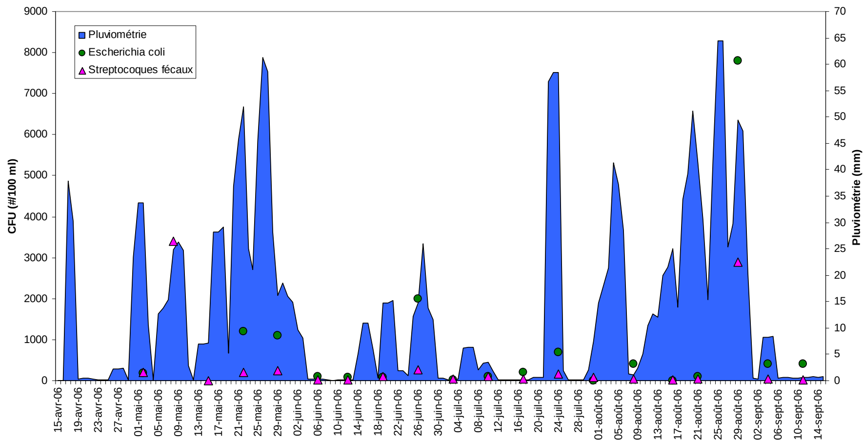
Figure 42 : évolution des paramètres bactériologiques et de la pluviométrie cumulée sur trois jours au cours de l'année 2006 Source des données : SPW/SETHY, 2009-2010
