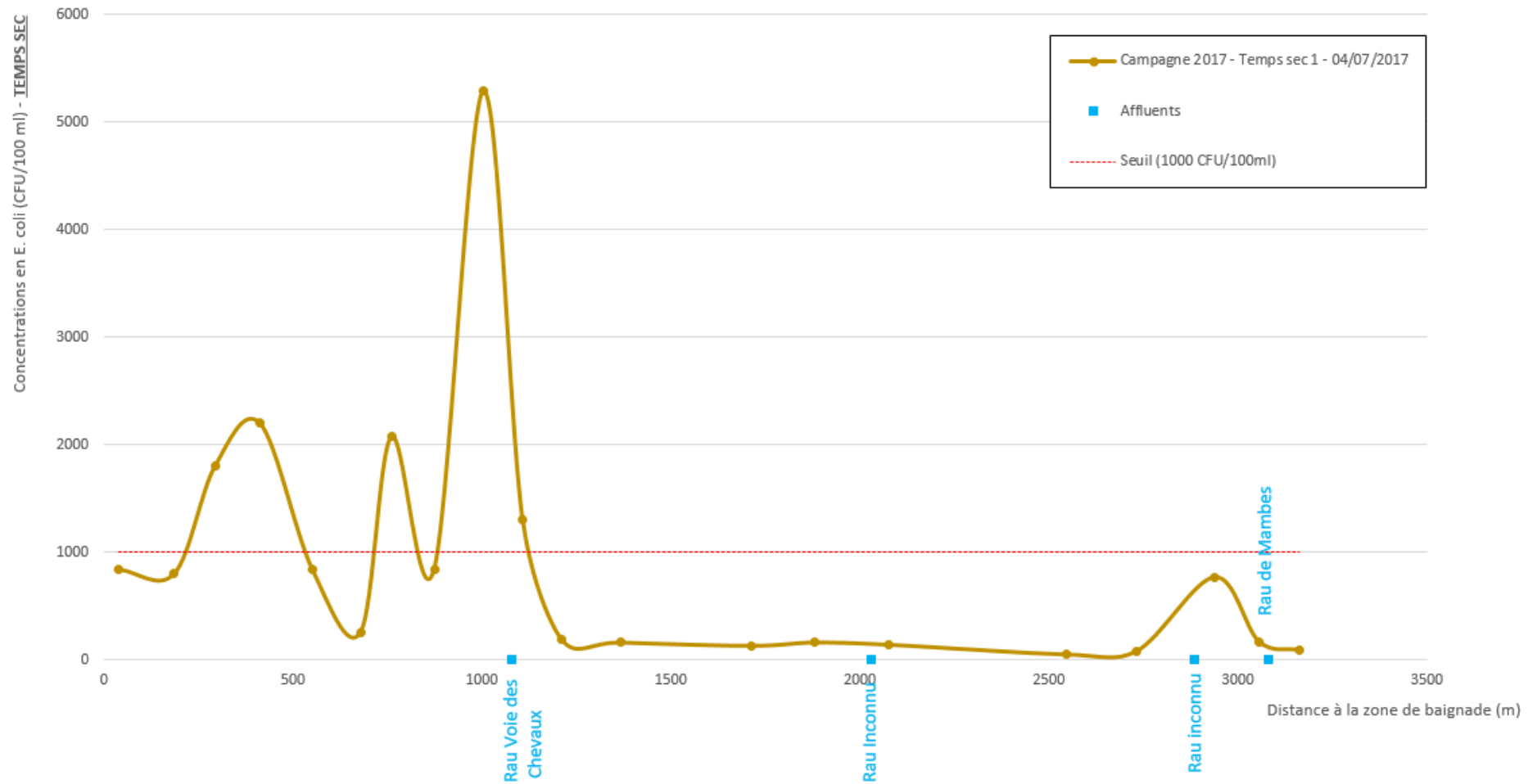
Figure 4 : profil longitudinal de l'évolution de la qualité bactériologique de la Semois sur la zone amont de Bouillon, lors de l'épisode « temps sec » du 04/07/2017. (Source des données : SPGE, 2017).
