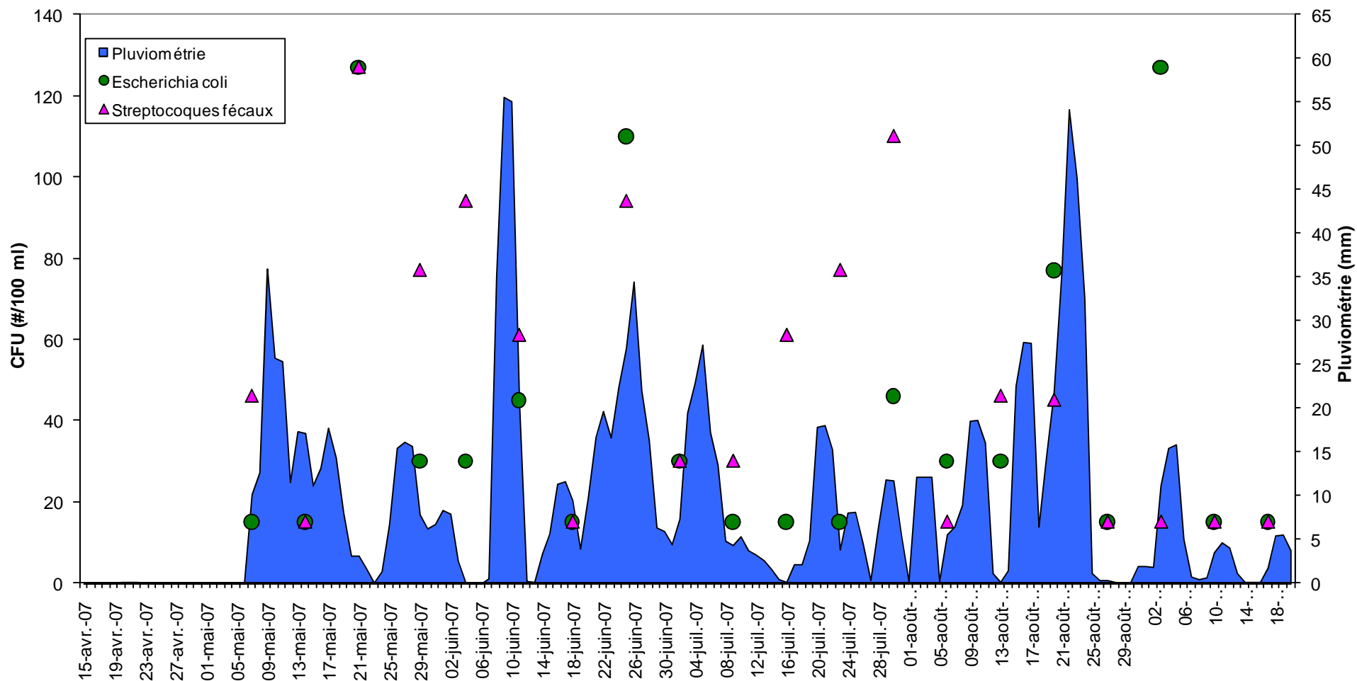
Figure 29: évolution des paramètres bactériologiques et de la pluviométrie cumulée sur trois jours au cours de l'année 2007.
