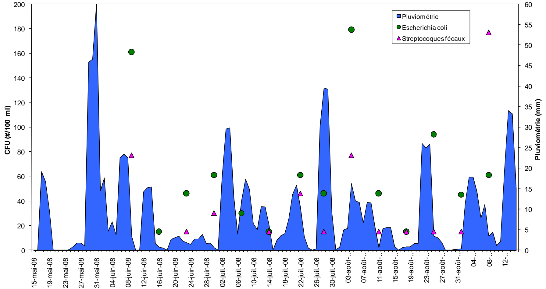
Figure 30 : évolution des paramètres bactériologiques et de la pluviométrie cumulée sur trois jours au cours de l'année 2008.
