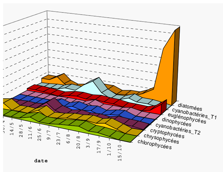
Figure 25 : phénologie du phytoplancton au lac de Chérapont Source : FUNPD, 2010
