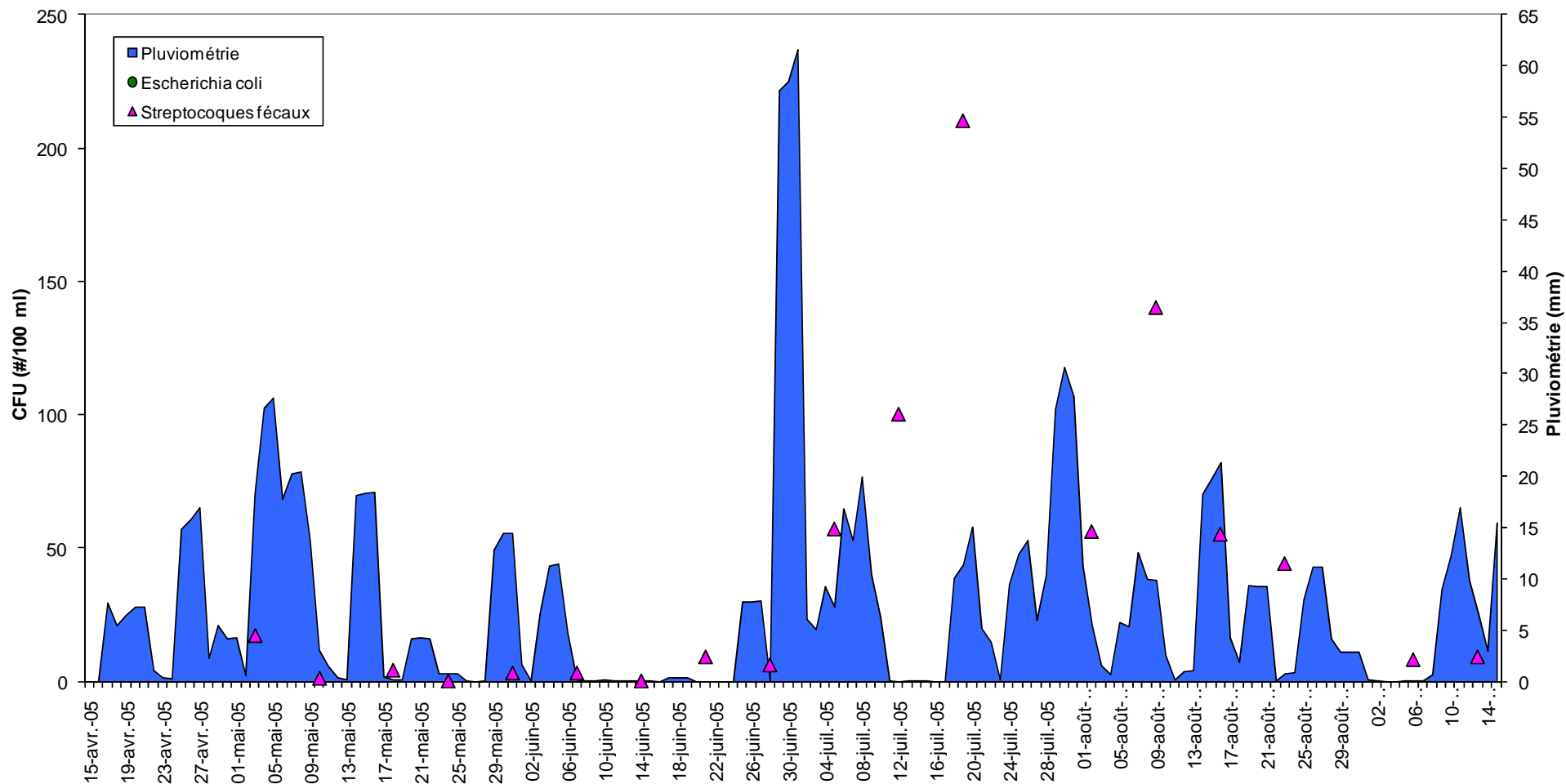
Figure 27: évolution des paramètres bactériologiques et de la pluviométrie cumulée sur trois jours au cours de l'année 2005. Source des données : SPW/SETHY, 2009-2010
