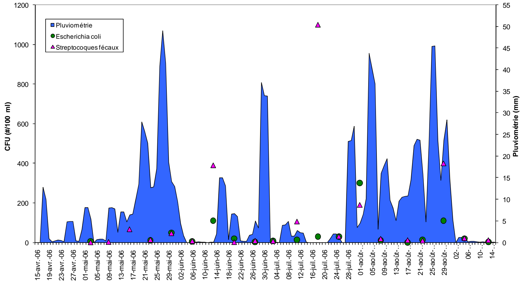
Figure 28 : évolution des paramètres bactériologiques et de la pluviométrie cumulée sur trois jours au cours de l'année 2006 Source des données : SPW/SETHY, 2009-2010
