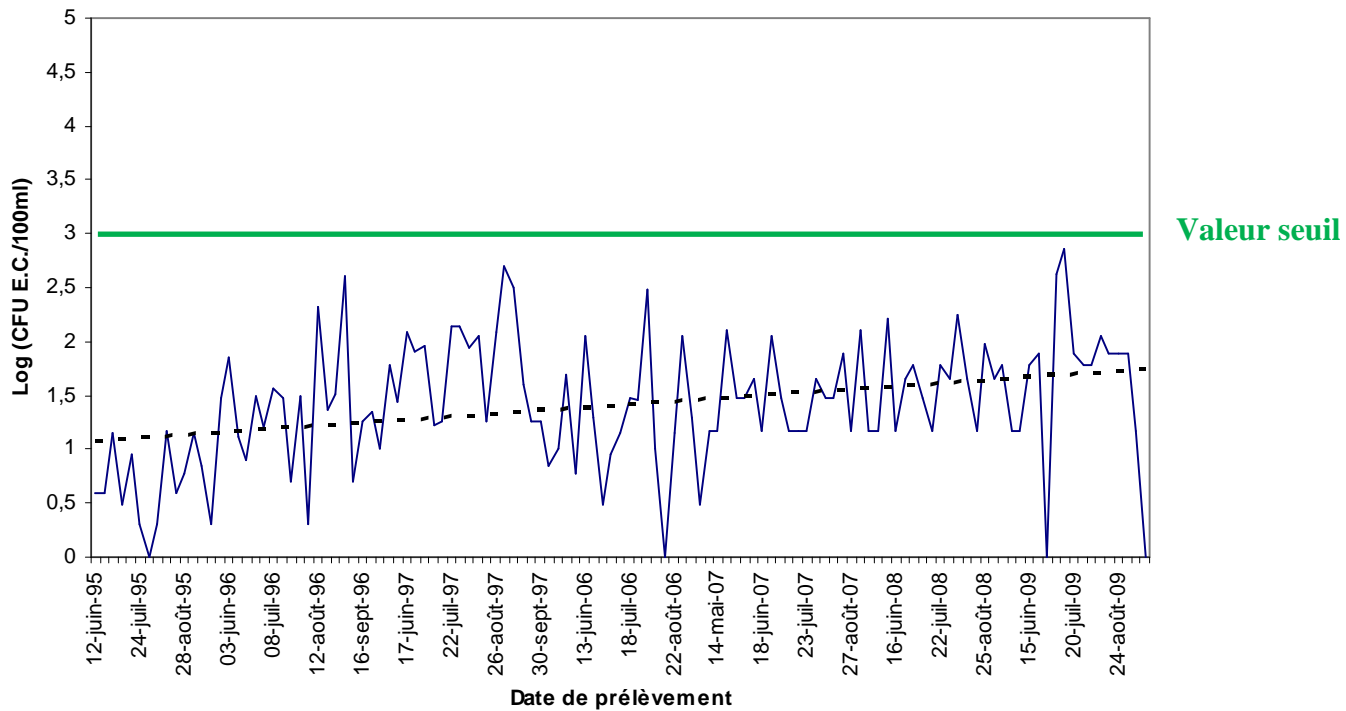
Figure 9: évolution des concentrations en E. coli (Log) sur la zone de baignade H06 entre 1995 et 1997 ainsi qu'entre 2006 et 2009 (n=119). Source : SPW-DGARNE-PROTECTIS, 2010
