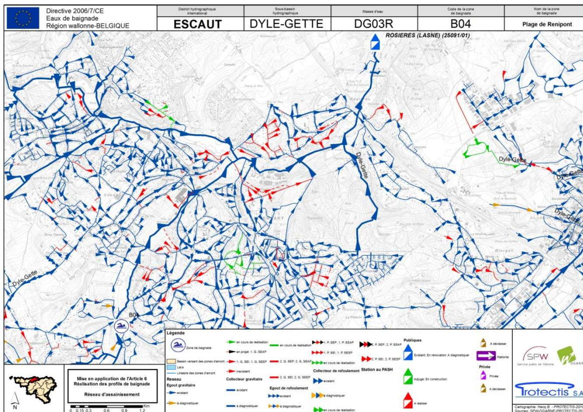
Figure 15: vue globale du réseau d'assainissement collectif autour de la zone de baignade B04 Source des données : SPGE, 2010
