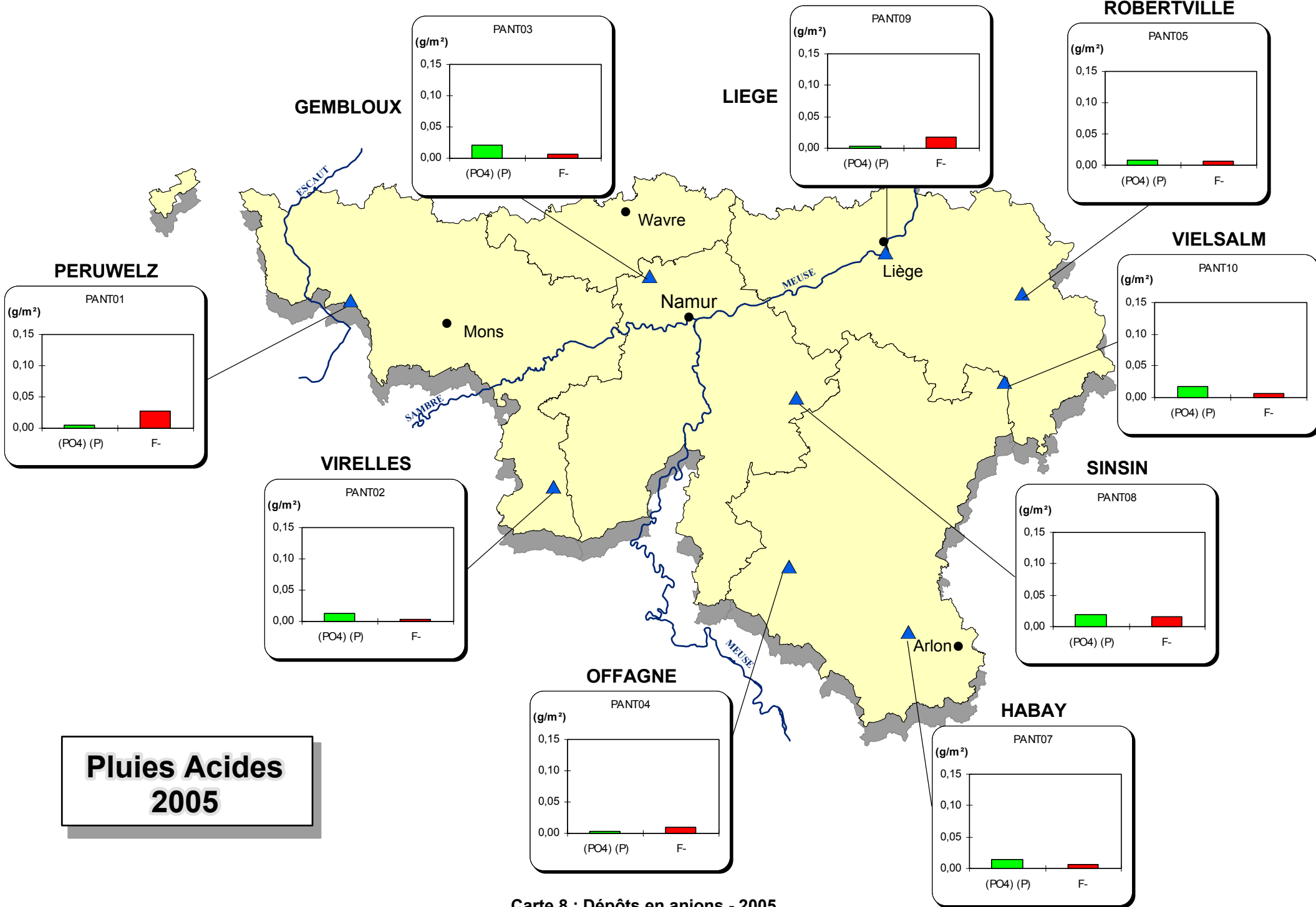
Carte 8 : Dépôts en anions - 2005
