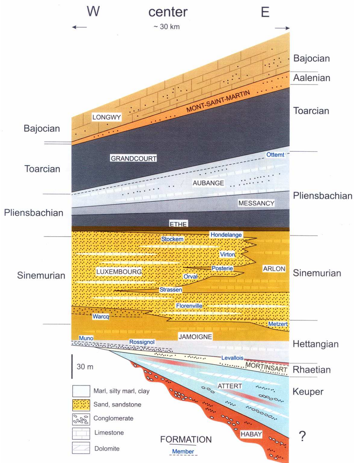
Figure 3.3 : Schéma lithostratigraphique général de la Lorraine belge (Bouvain et al. 2001)
