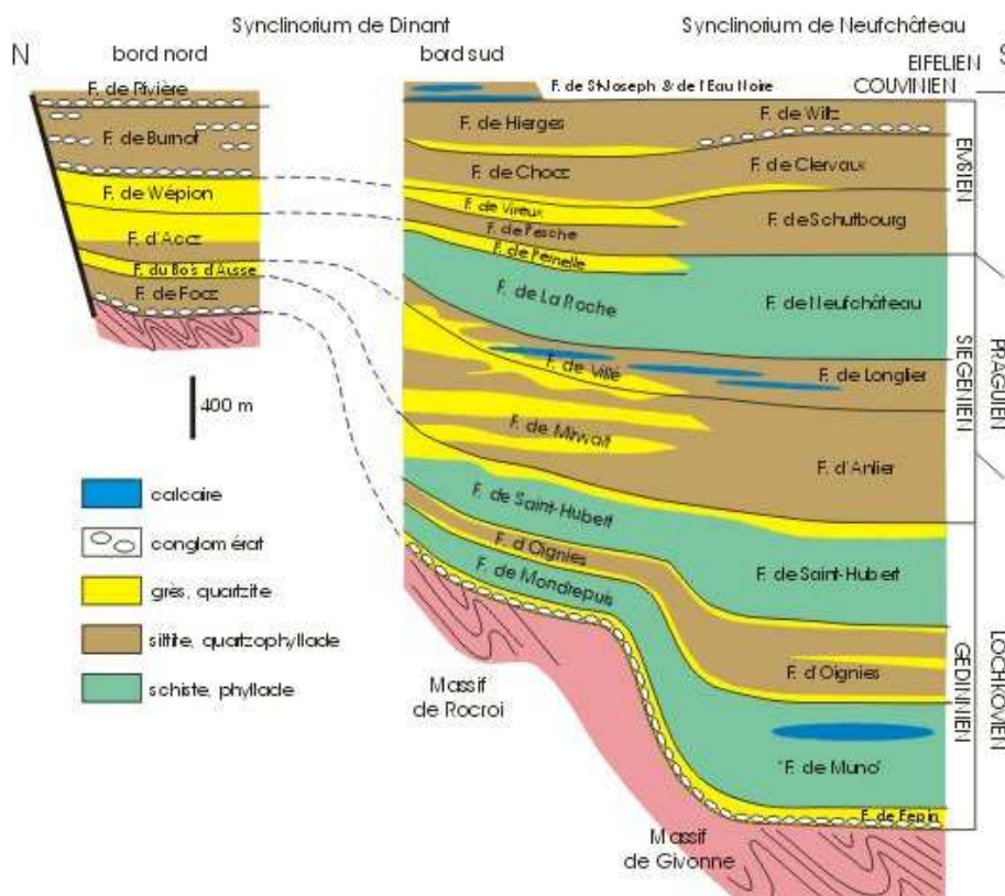
Figure 3.2 : Transect Nord-Sud dans les Synclinoiria de Dinant et de Neufchâteau, durant le dépôt du Dévonien Inférieur (Boulvain et Pingot, 2004)
